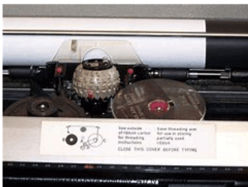
Detalj av IBM Composer med skrivkula
