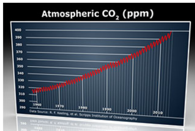
Keeling-kurvan
