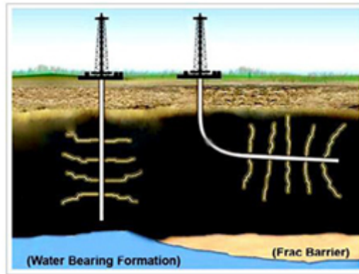
Fig. 2 Horisontella borrhål
